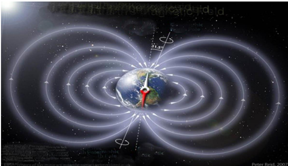
Hình vẽ minh họa về trường điện từ của Trái Đất
