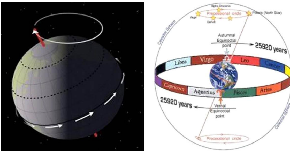
Hình vẽ mô tả sự tiến động thẳng hàng của trục Trái Đất
