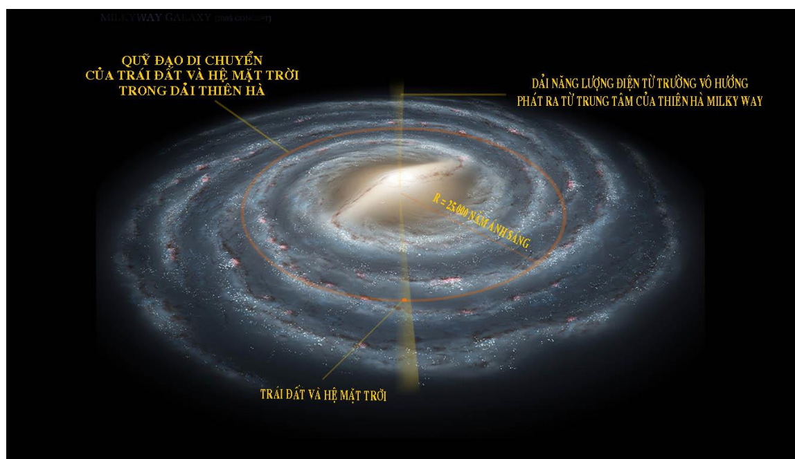
Hình ảnh mô tả về sự Chuyển Đổi Thiên Hà của Trái Đất và Hệ Mặt Trời
